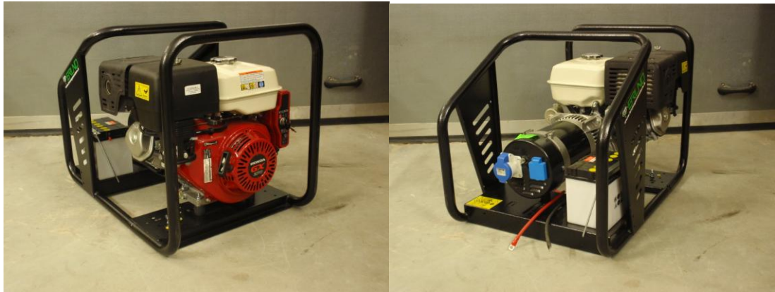
5 kVA (4 kW) Bruno (Itālija) elektrostacija, 230 V, Honda benzīna motors, rokas spoles un elektriskais starts, 1.5 l/h degvielas patēriņš pie 75% slodzes, 6 l degvielas tvertne. Cena 700,- LVL ar PVN
