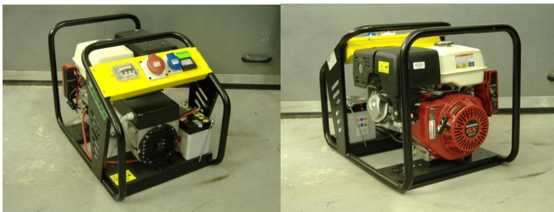
6.5 kVA (5.2 kW) Bruno (Itālija) elektrostacija, 230/400 V, Honda benzīna motors, rokas spoles un elektriskais starts, 1.5 l/h degvielas patēriņš pie 75% slodzes, 6 l degvielas tvertne. Cena 850,- LVL ar PVN
