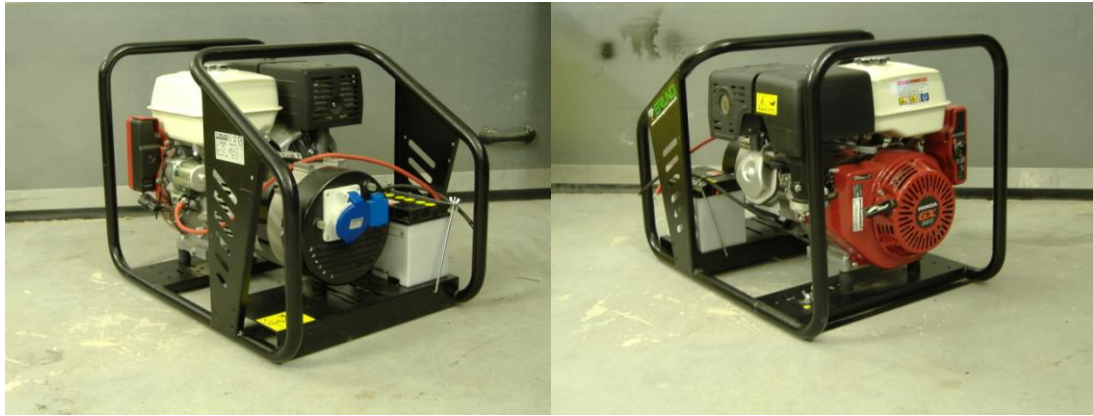
7.5 kVA (6 kW) Bruno (Itālija) elektrostacija, 230 V, Honda benzīna motors, rokas spoles un elektriskais starts, 1.9 l/h degvielas patēriņš pie 75% slodzes, 6 l degvielas tvertne. Cena 850,- LVL ar PVN
